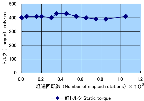
OTLV6-4000C 信頼性試験データ (50 rpm. 連続) OTLV6-4000C Reliability test data (at 50rpm.)
