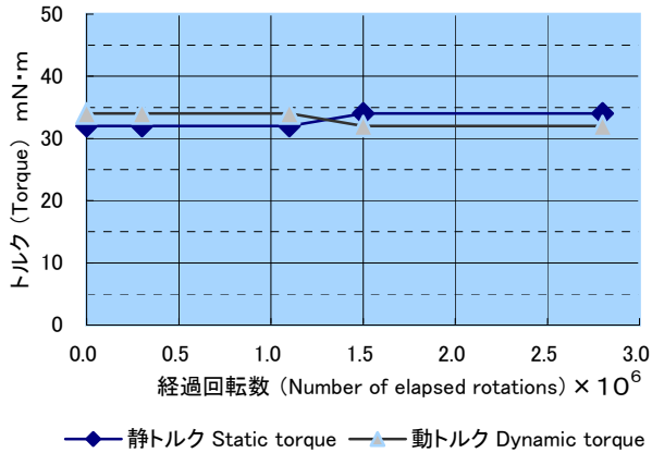
OTLV6-300B 信頼性試験データ (150 rpm. 連続) OTLV6-300B Reliability test data (at 150rpm.)
