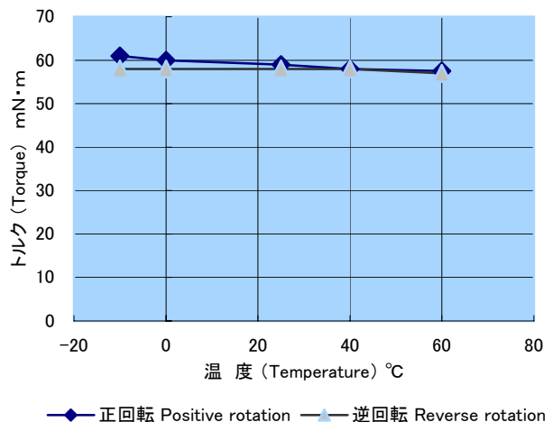
OTLV6-600B 環境特性 (湿度 90%RH) OTLV6-600B Environmental characteristics (humidity 90%RH)
