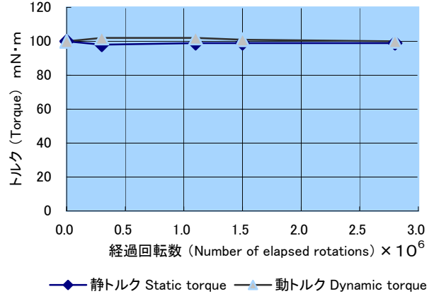
OTLV6-1000B 信頼性試験データ (150 rpm. 連続) OTLV6-1000B Reliability test data (at 150rpm.)
