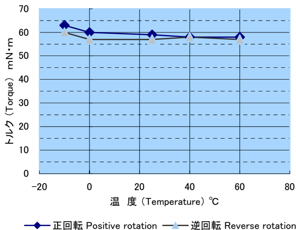
OTLV6-600B 環境特性 (湿度 30%RH) OTLV6-600B Environmental characteristics (humidity 30%RH)
